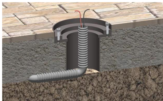
Cassa a filo pavimento su fondo drenante. Fori di fissaggio corpo perpendicolari all'emissione luce
