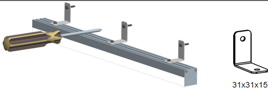
Fissaggio tramite Staffa ST.031.031 con viti diametro max. 3mm
