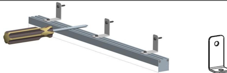
Fissaggio tramite staffa ST.031.014 con viti diametro max. 3mm
