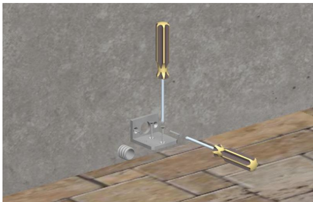
Posizionare e fissare staffa con viti adatte al supporto. Viti non fornite
